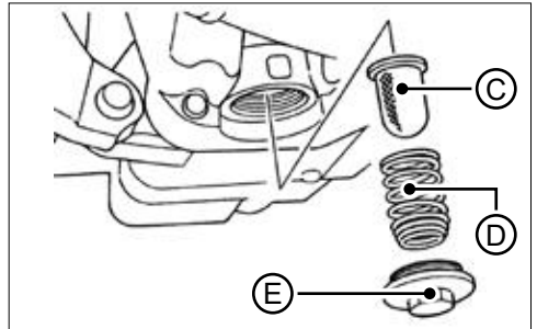
C Ölfiltersieb
